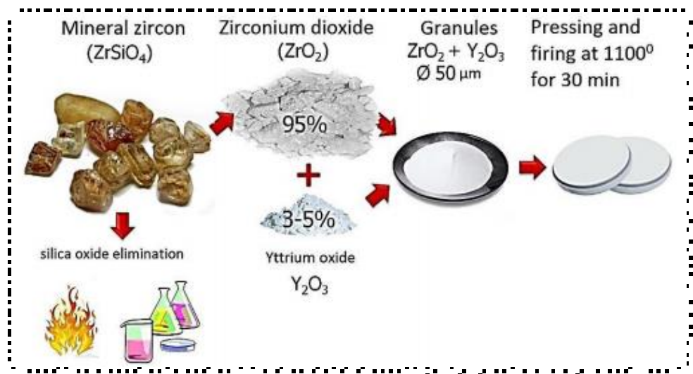
Slika 35. Shematski prikaz proizvodnje itrijevim dioksidom parcijalno stabiliziranog cirkonija. (Osnovni koncept ilustracije preuzet iz 75. Individualizirao i uredio autor.)
