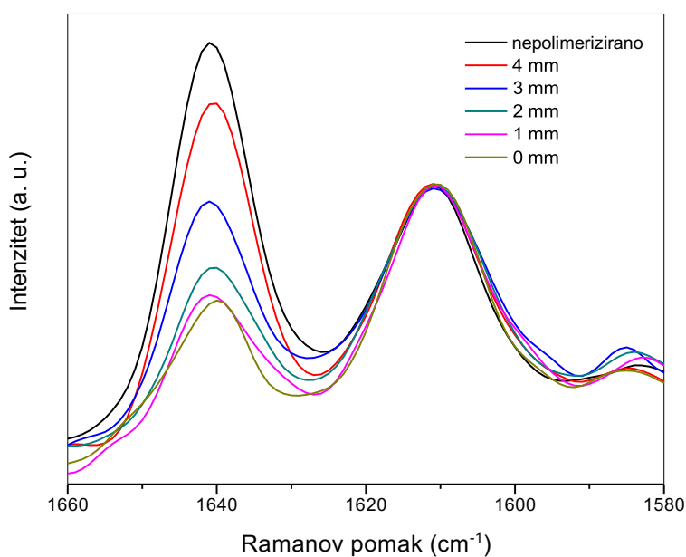
Slika 19. Dio Ramanovog spektra koji se koristi za mjerenje stupnja polimerizacije kod kompozitnih materijala. Nakon normiranja spektara na referentnu vrpce na 1610\text{ cm}^{-1} , razlike u intenzitetu vrpce na 1640\text{ cm}^{-1} ukazuju na smanjenje učinkovitosti polimerizacije s povećanom debljinom sloja kompozitnog materijala. Preuzeto i prilagođeno iz (126).
