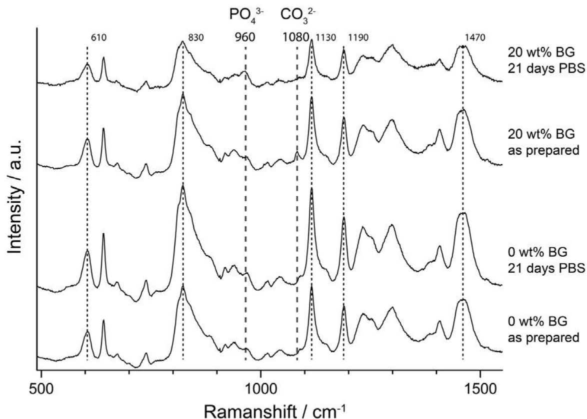
Slika 20. Ramanovi spektri snimljeni s površine bioaktivnih materijala koji na svojoj površini precipitiraju hidroksiapatit. Promjene intenziteta vrpce na 960 \text{ cm}^{-1} ukazuju na pojavu hidroksiapatita na površini materijala nakon imerzije u vodenom mediju. Preuzeto iz (127).
