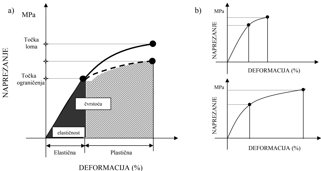
Slika 2. Tipična krivulja naprezanje-deformacija. Površina ispod krivulja pokazuje količinu elastičnosti i čvrstoće (a). Krivulje naprezanje-deformacija za kompozitni materijal i akrilnu plastiku. Oba materijala pokazuju istu elastičnosti ali akrilna plastika je mnogo
