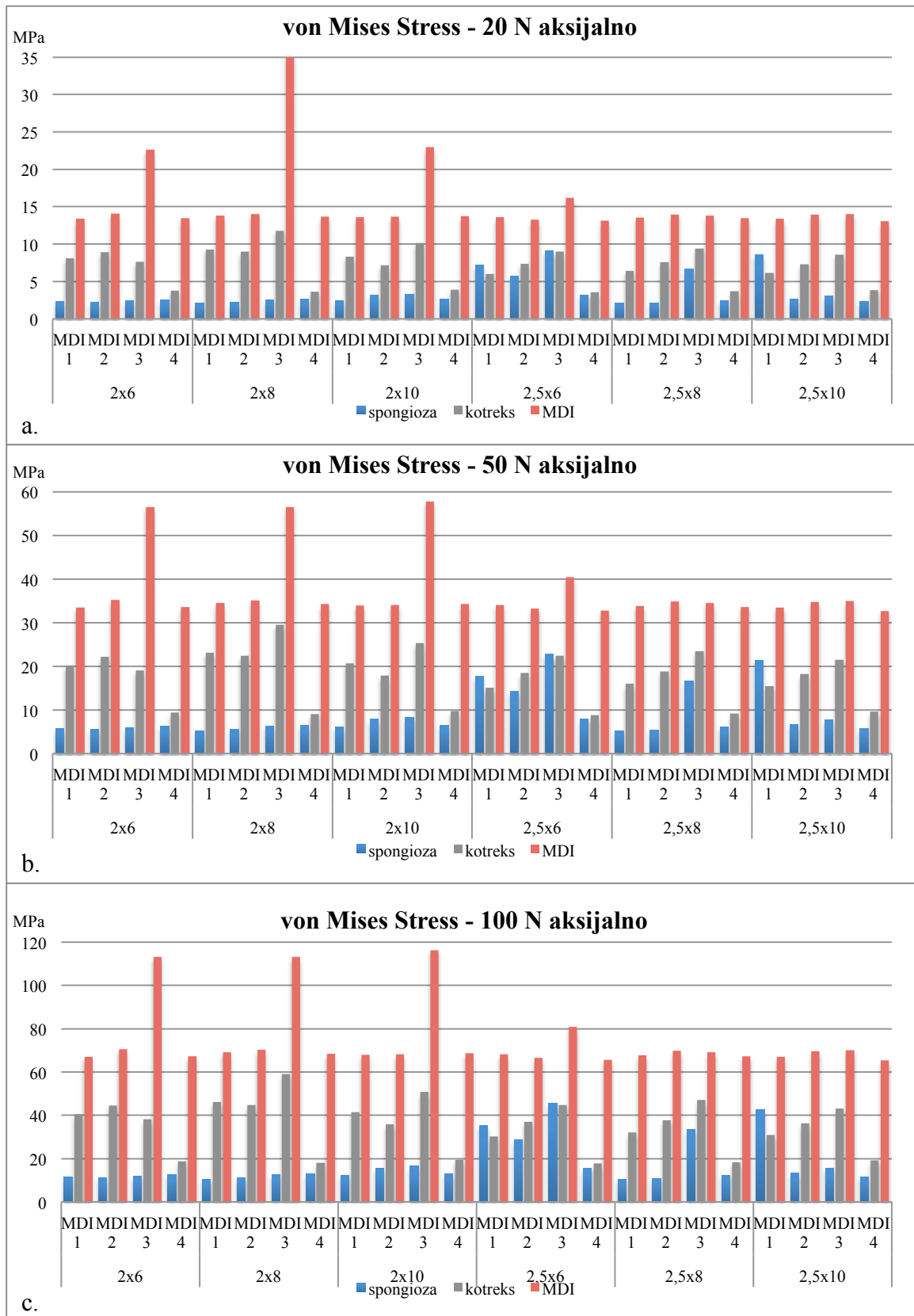
Slika 39. Grafički prikaz iznosa maksimalnog stresa (von Mises Stress) kod aksijalnog opterećenja na površini mini dentalnog implantata i na kontaktnoj površini spongioze i korteksa: a. 20 N; b. 50 N; c. 100 N
