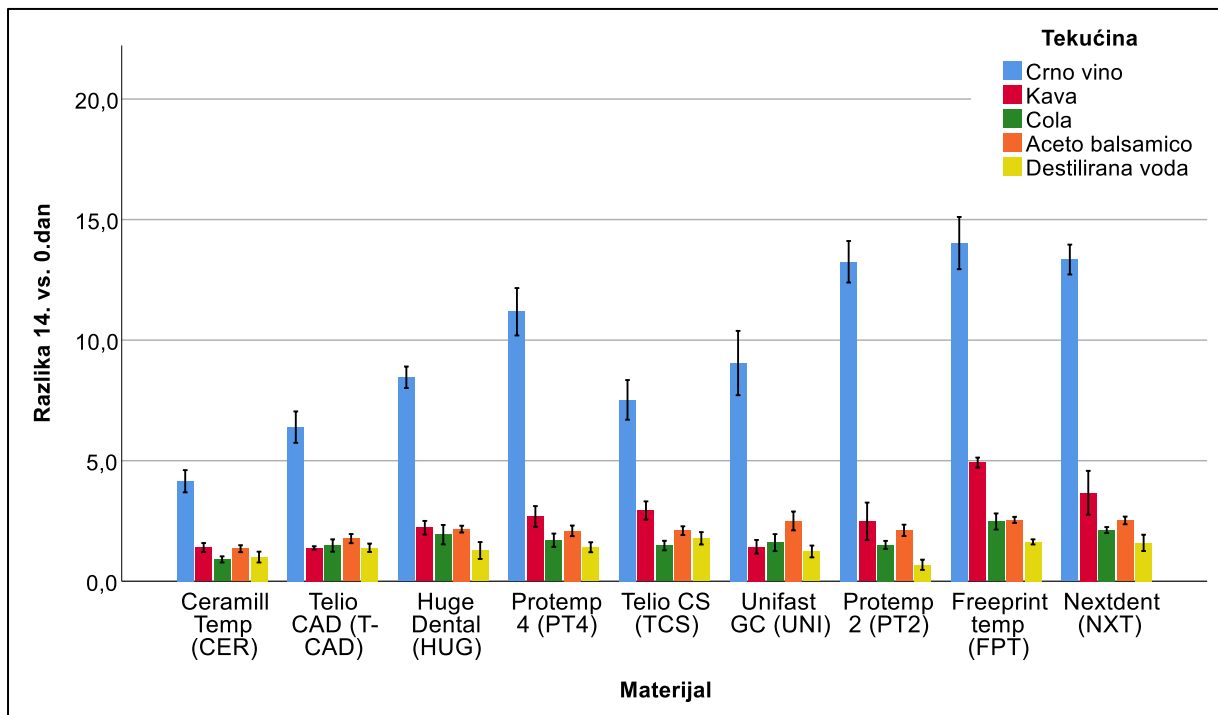
Slika 7. Usporedba \Delta E vrijednosti (promjena boje) za testirane materijale u različitim otopinama nakon 14 dana
