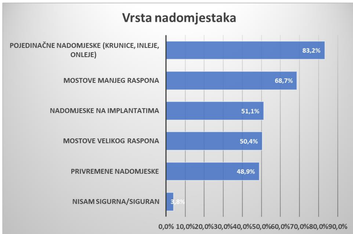
Slika 4. Najčešće izrađivani nadomjestci primjenom CAD/CAM tehnologije.
