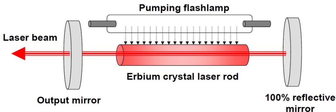
Slika 3. Pojednostavljena konfiguracija erbijskog lasera (preuzeto iz 53)
