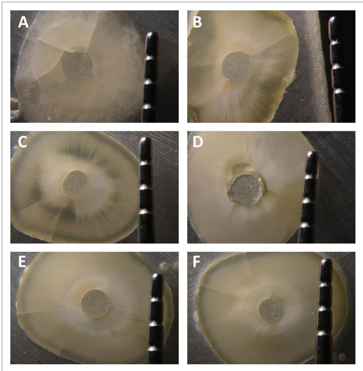
Slika 22. Primjeri vrste popuštanja uzoraka. Slike A, C, E i F prikazuju adhezivni tip popuštanja. Slike B i D prikazuju mješviti tip popuštanja.
