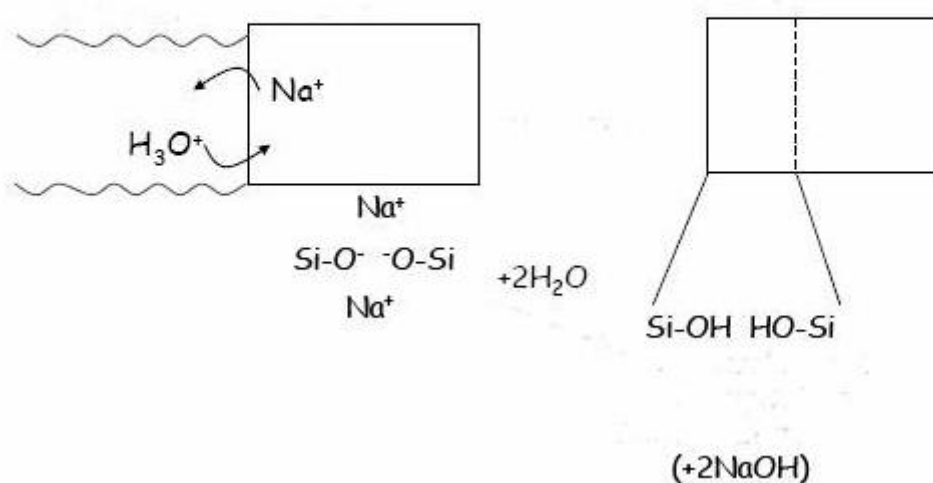
Slika 52. Reakcija selektivnog izluživanja (preuzeto iz 183)
