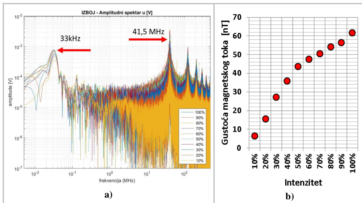
Slika 53. Magnetsko polje: a) prikaz amplitudnog spektra izboja kroz zrak (crvene strelice: frekvencijske komponente signala u području 33 kHz i iznad 40 MHz), b) izmjerene vrijednosti gustoće magnetskog toka B [nT] na frekvenciji 41,5 MHz kao funkcija intenziteta
