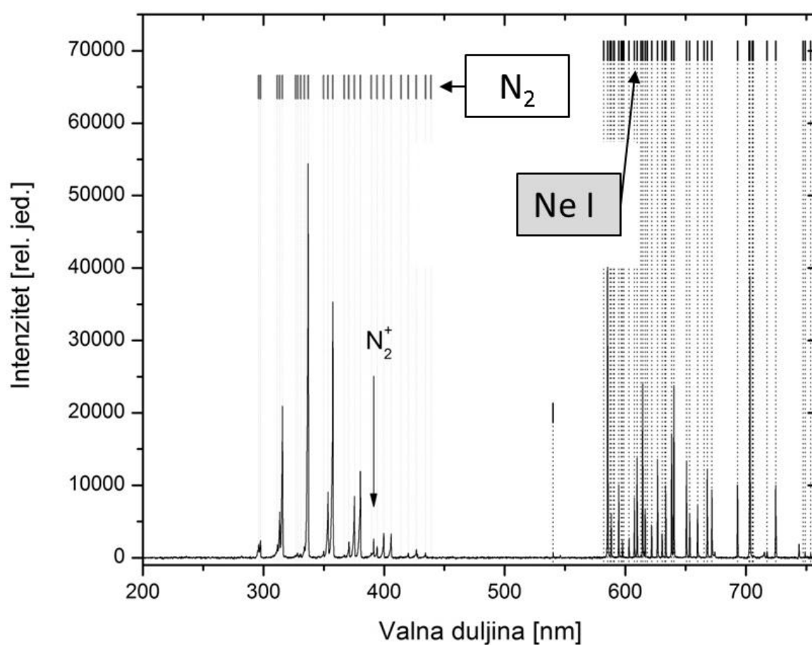
Slika 44. Emisijni spektar zabilježen prilikom izboja na malu površinu žice (površine 0,8 \text{ mm}^2 ) u kojem se uz spektralne linije neutralnog atoma neona ( \text{Ne I} ) i molekule dušika ( \text{N}_2 ) javlja i linija iona dušikove molekule ( \text{N}_2^+ )
