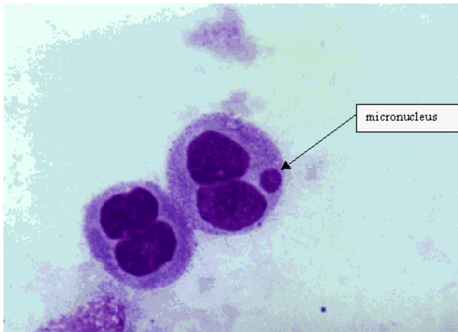
Slika 30. Formiranje mikronukleusa.
