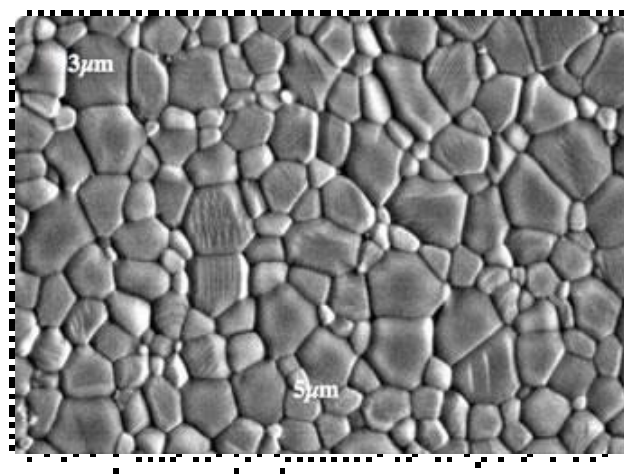
Slika 36. Mikrostruktura \text{Al}_2\text{O}_3 keramike. (Osnovni koncept ilustracije preuzet iz 105. Individualizirao i uredio autor.)
