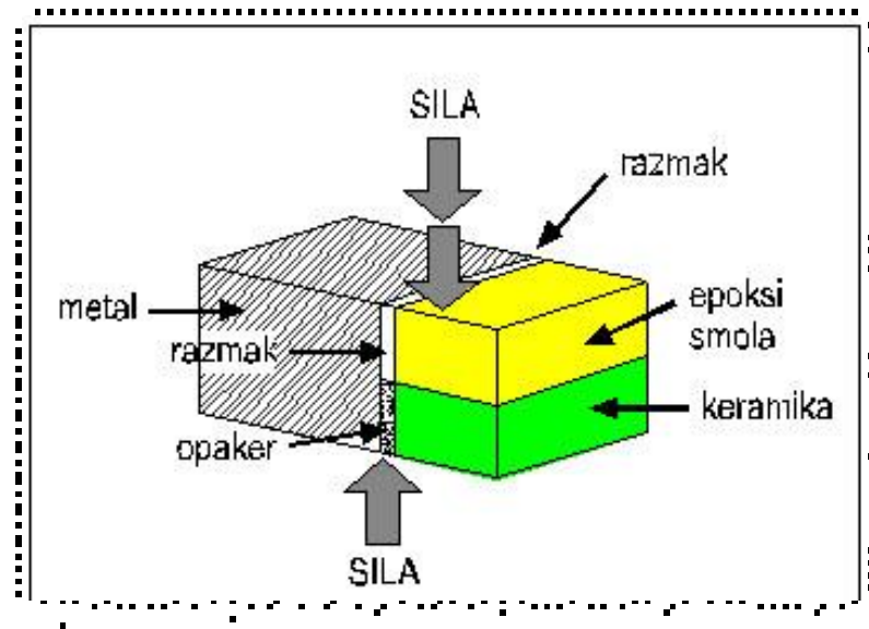
Slika 43. Pravokutni međuspojni smični test po Schmitzu i Schulmeyeru. (Osnovni koncept ilustracije preuzet iz 131. Individualizirao i uredio autor.)
