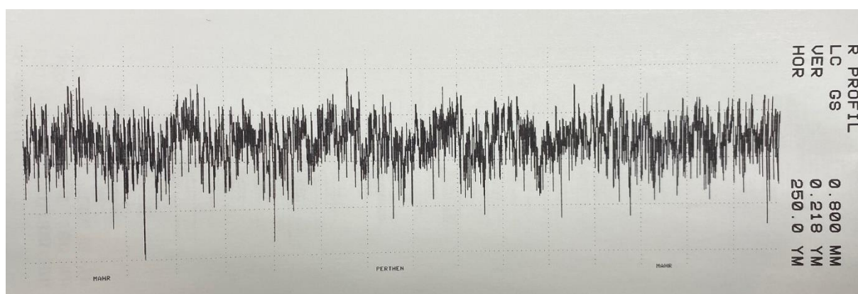
Slika 77 a. Hrapavost skupine tretirane silanom – grafički prikaz (uzorak 1).
