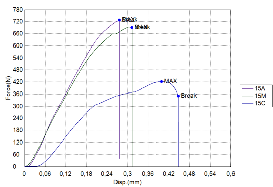
Slika 34. Dijagram sila-pomaka za uzorak 15 – Reciproc Blue grupa.
