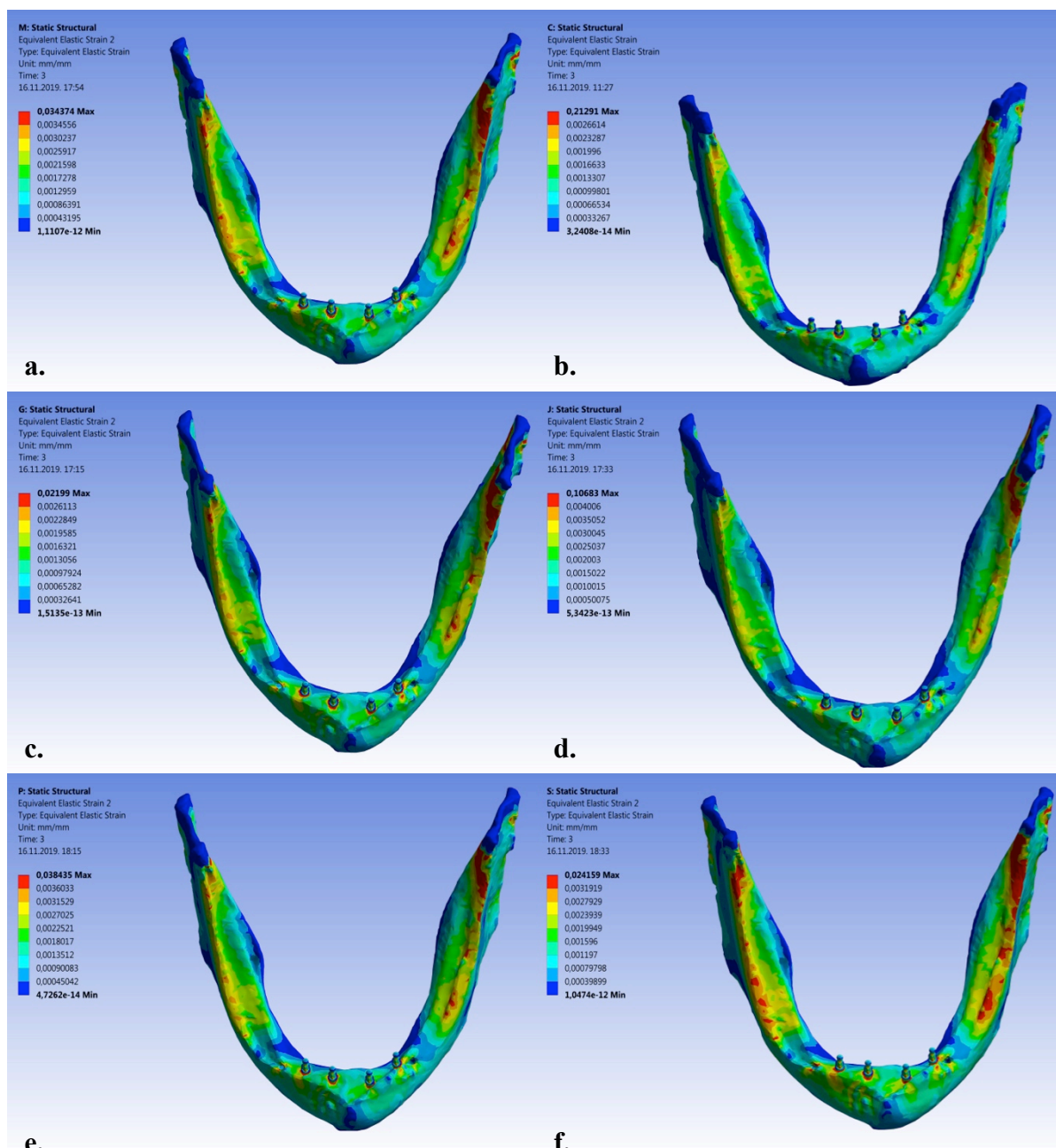
Slika 32. Prikaz raspodjele naprezanja (von Mises Strain) kod kosog ( 45^\circ ) opterećenja sa 100 N po mini dentalnom implantatu: a. 2 x 6; b. 2,5 x 6; c. 2 x 8; d. 2,5 x 8; e. 2 x 10; f. 2,5 x 10
