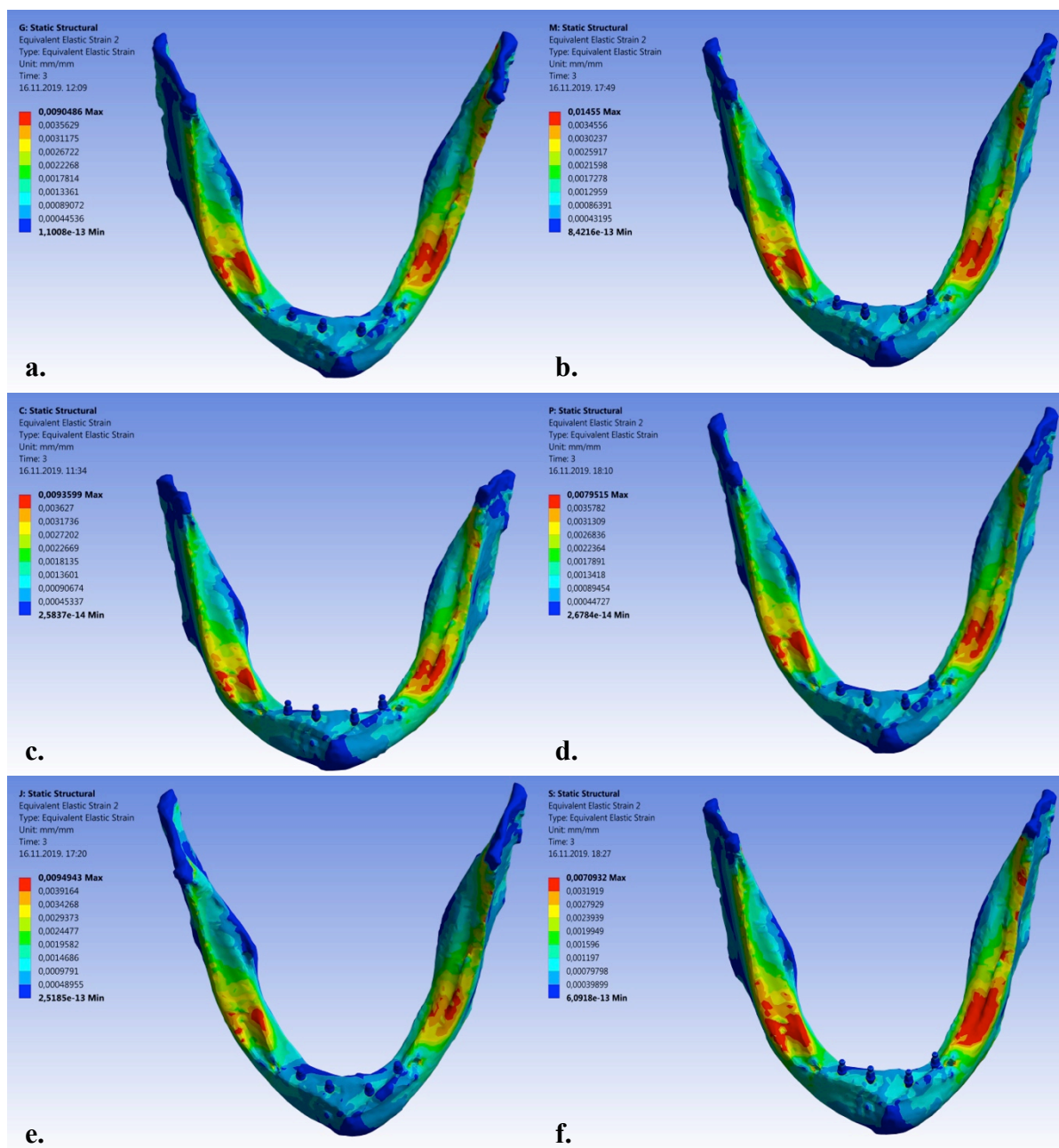
Slika 28. Prikaz raspodjele naprezanja (von Mises Strain) kod aksijalnog opterećenja sa 100 N po mini dentalnom implantatu: a. 2 x 6; b. 2,5 x 6; c. 2 x 8; d. 2,5 x 8; e. 2 x 10; f. 2,5 x 10
