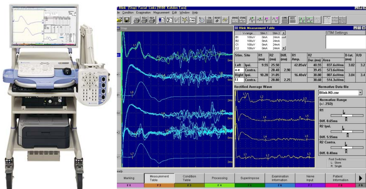
Slika 60. Elektromiografski aparat MEB 2300 (Nihon Kohden).
