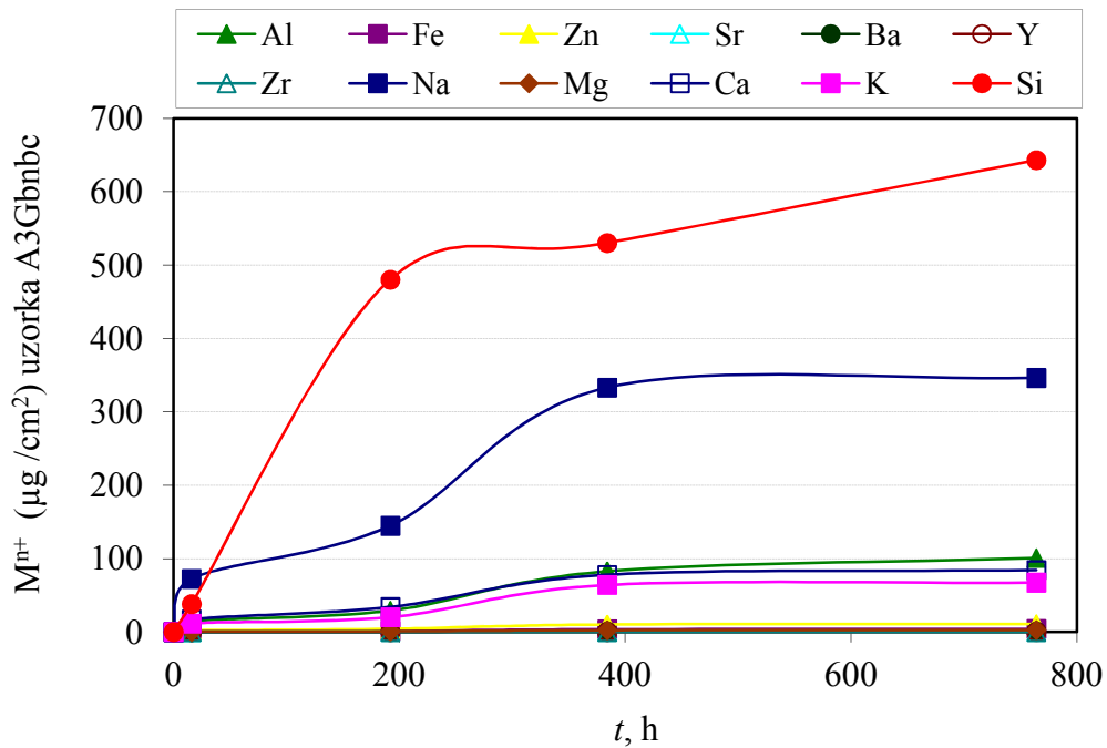
Slika 43. Ovisnost količine eluiranih iona iz zubne keramike (uzorak A3G) o vremenu izloženosti u 4%-tnoj CH 3 OOH otopini.
