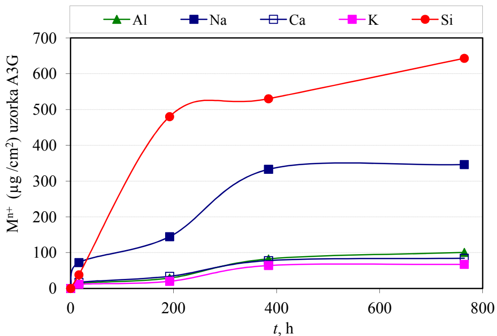
Slika 44. Usporedba količine eluiranih iona Al 3+ , Na + , Ca 2+ , K + i Si 4+ iz zubne keramike (uzorak A3G) u 4%-tnoj CH 3 OOH otopini kao funkcija vremena izloženosti.
