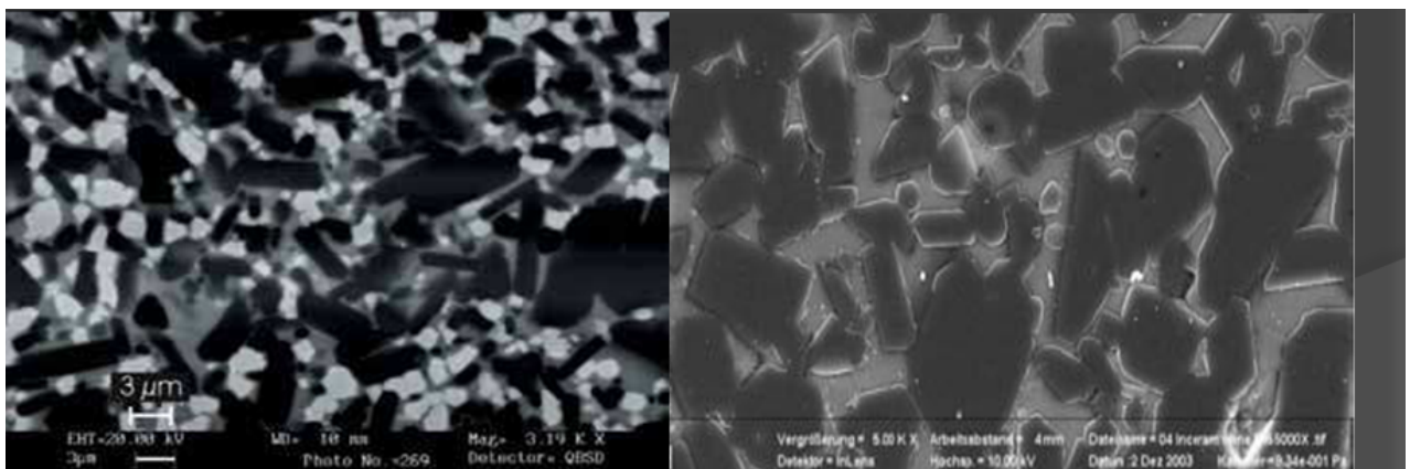
Slika 15. SEM-Slika VITA In-Ceram® ZIRCONIA. Preuzeto iz (49).
