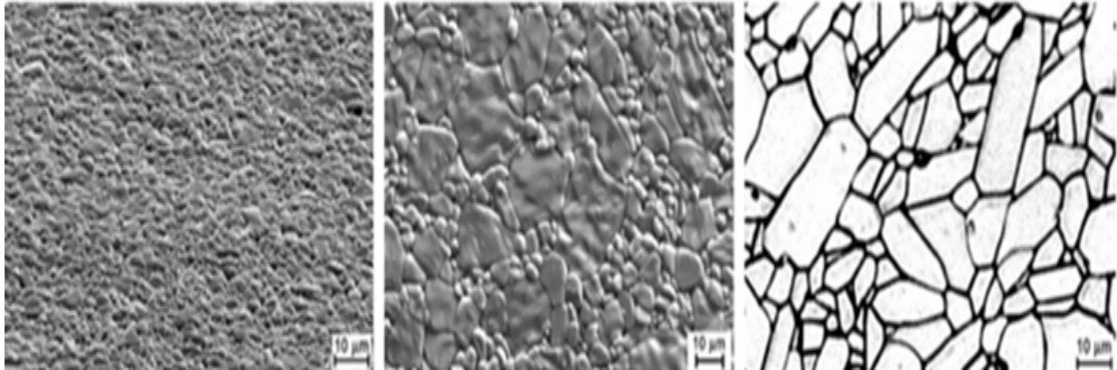
Slika 14. Mikrostruktura aluminij-oksidge keramike. Preuzeto iz (46).
