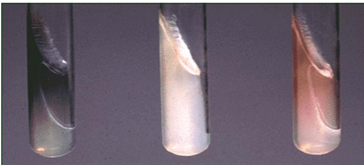
Slika 6. Pigmenti koje stvara P. aeruginosa – fluorescein, piorubin i piocianin koji su važni čimbenici virulencije. Izvor: KBC Zagreb
