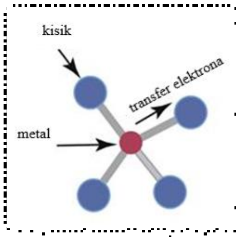
Slika 3. Ionska veza.
