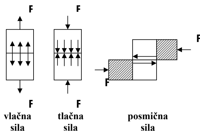
Slika 1. Vrste naprezanja
