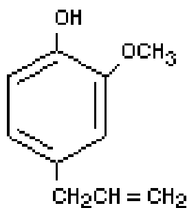
Slika 1. Strukturna formula eugenola
