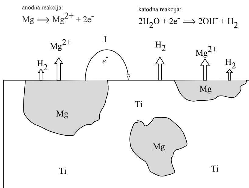
Slika 58. Shema mikrogalvanske korozijske na površini eksperimentalnog Ti-Mg kompozita tijekom statičkog testa uranjanja.
