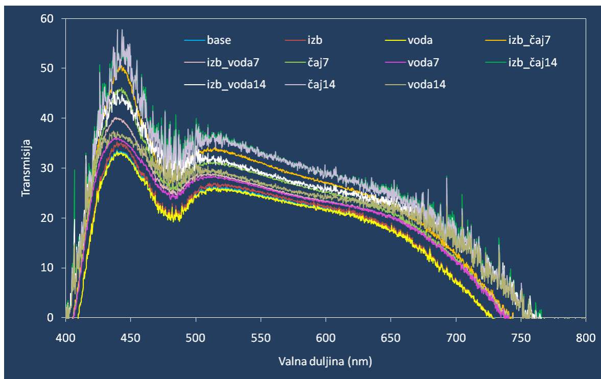
Slika 18. Rezultati transmisije za EQUIA u vidljivom dijelu spektra (400-800 nm)
