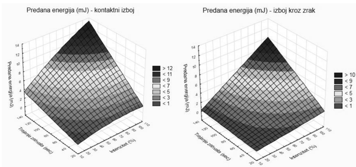
Slika 67. Predikcija predane energije (mJ) prema intenzitetu i trajanju zahvata kvadratnim regresijskim modelom za kontaktini izboj i izboj kroz zrak
