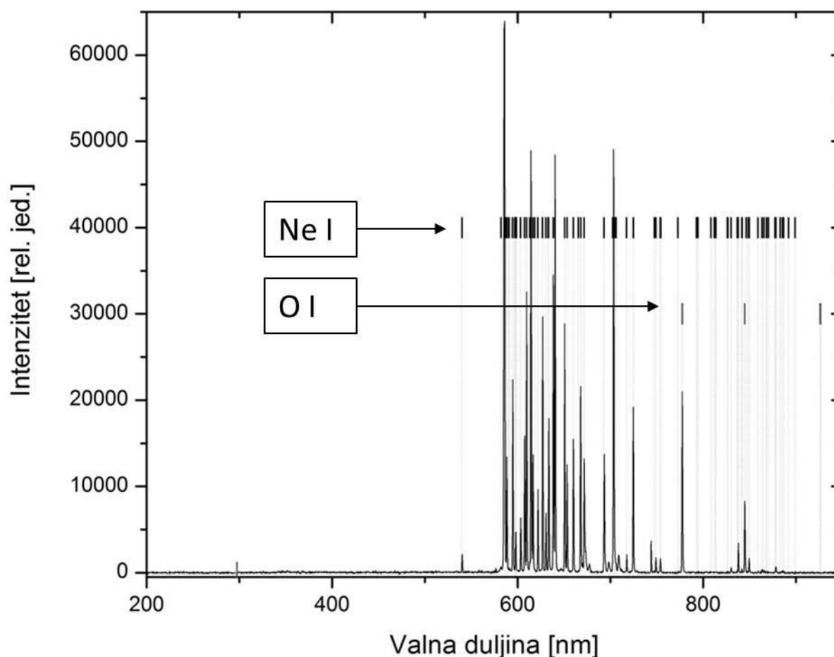
Slika 42. Emisijski spektar elektrode mjerena optičkim vlaknom izravno usmjerenim u aktivnu površinu elektrode. Bilježe se atomske linije neona i linije atoma kisika (prikazano područje od 200 do 950 nm)
